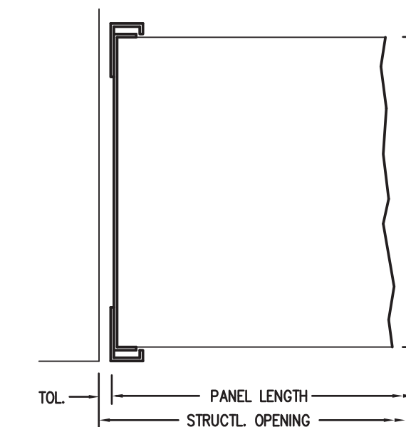
877. JAMB DETAIL
