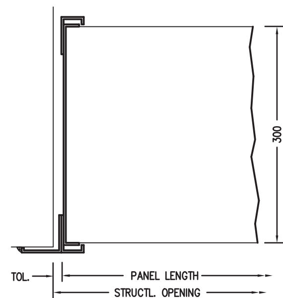
872. JAMB DETAIL
